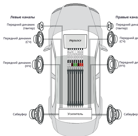
Подключение с использованием только RCA-выходов
